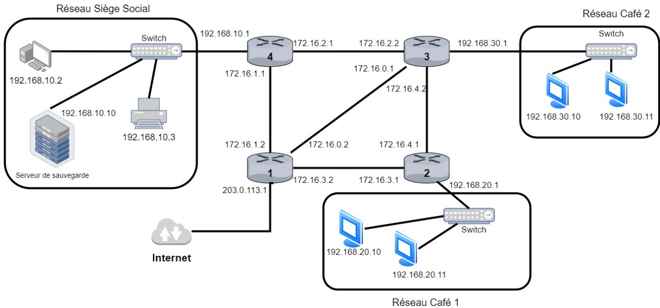
Figure 1. Schéma d'une partie du réseau
