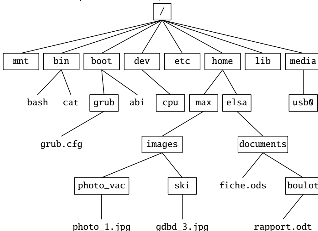
Figure 1 : Arborescence des fichiers
